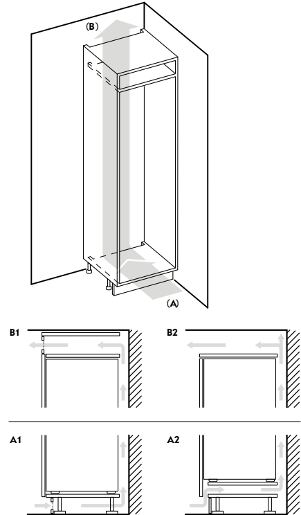
Suggerimenti di installazione per l'aerazione dell'apparecchio
