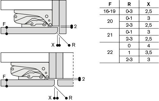
Dimensioni raccomandate per cerniere piate
