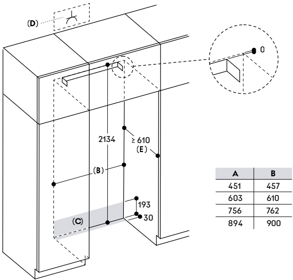
A: Larghezza dell'apparecchio B: Larghezza della nicchia C: Area di installazione per la connessione dell'acqua D: Spina E: Profondità della nicchia
