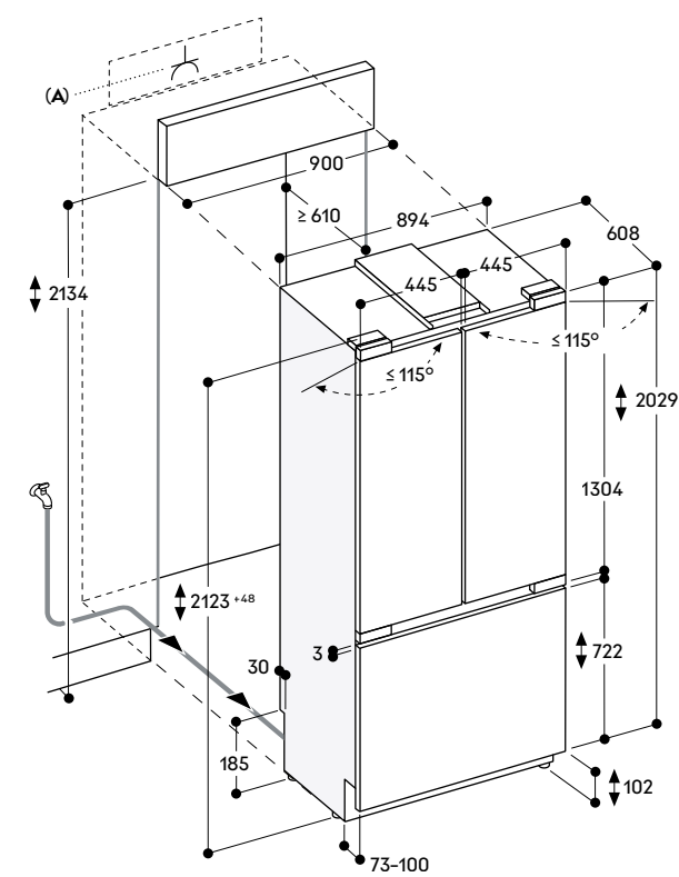
A: Presa La dimensione massima del pannello porta è basata su una tolleranza di 3 mm. L'altezza dello zoccolo può essere ridotta a 50 mm.
