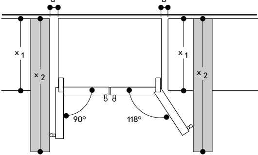
Angolo di apertura delle porte
