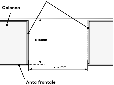
Nicchia. Taglio orizzontale
