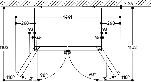
Distanze per l'apertura delle porte
